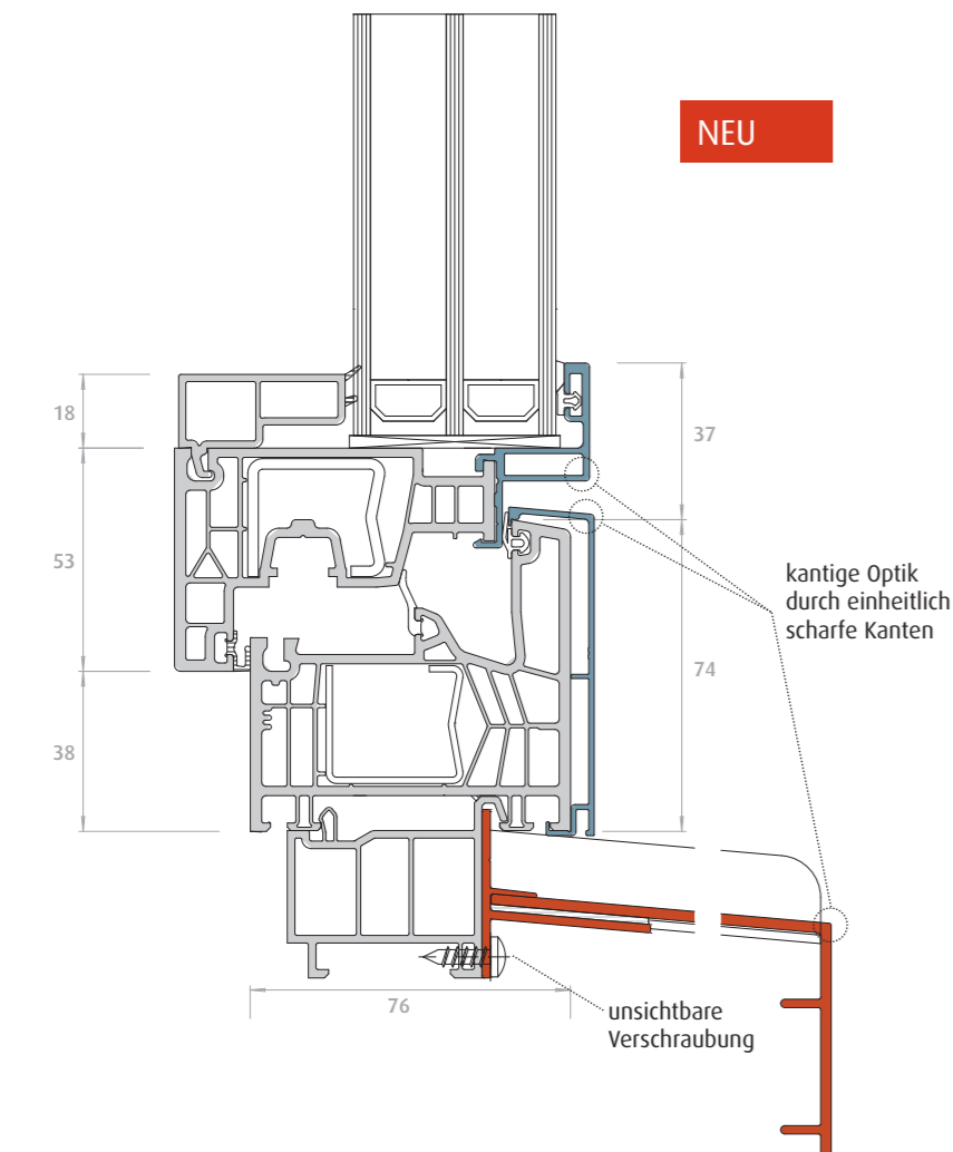
ip-Fensterbank 190 mm Ausladung
