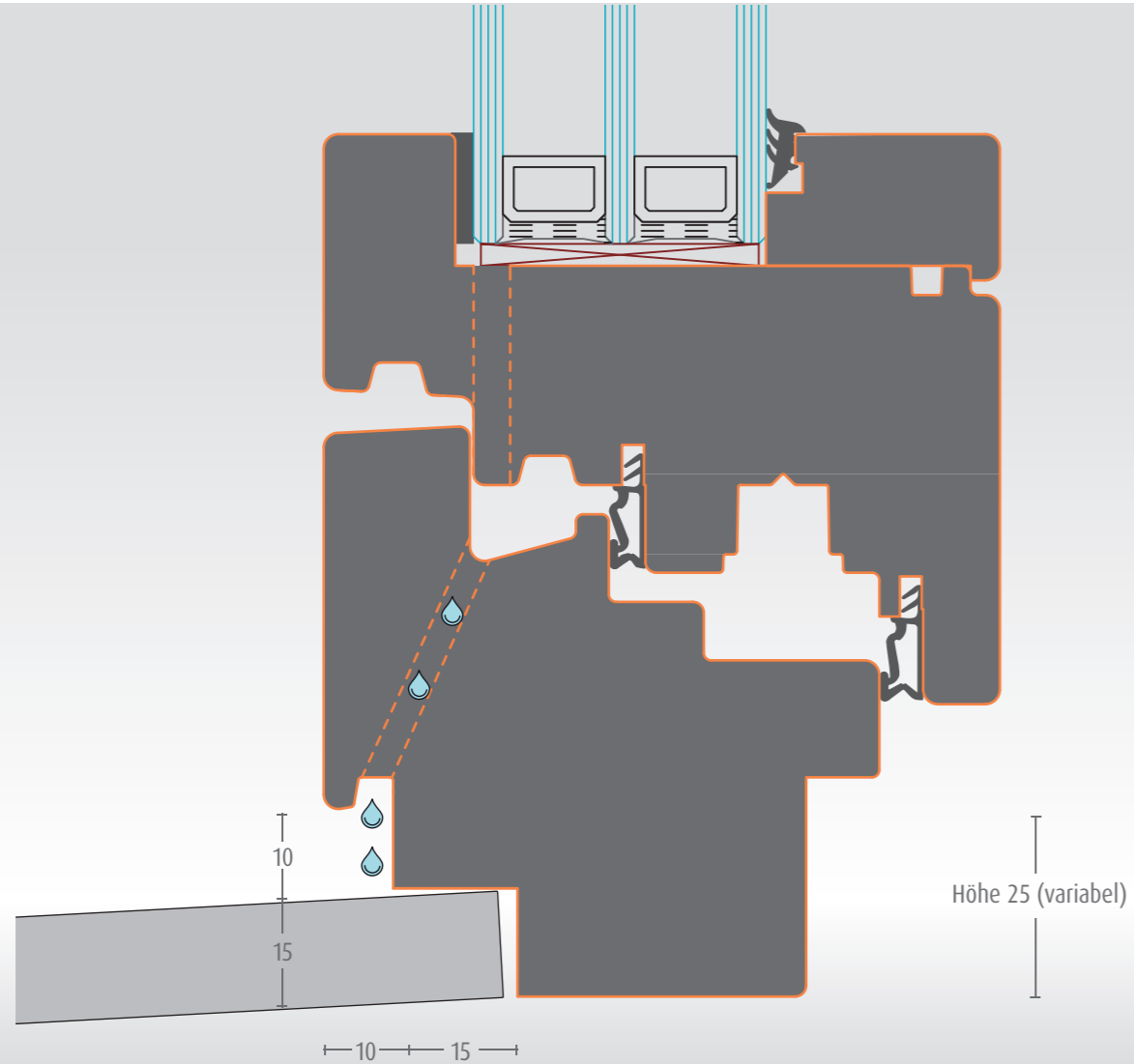
Steinbankanschluss
