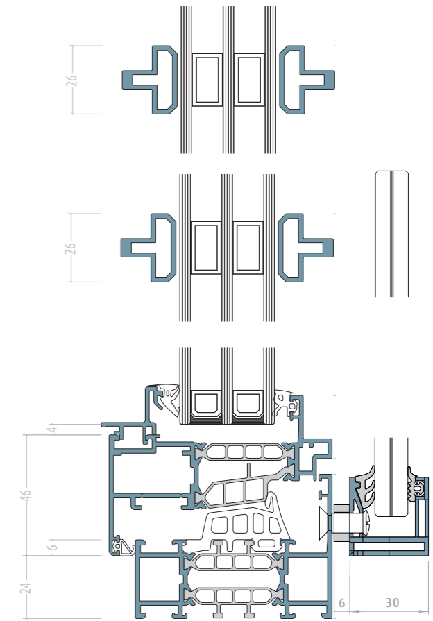
Glasabsturzicherung Typ1 und breiter Rahmen
