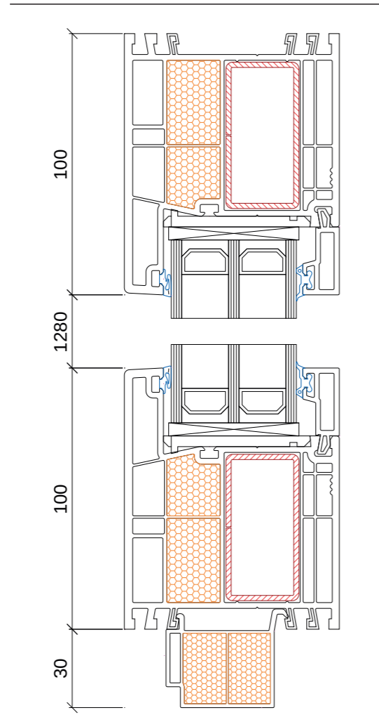
Festverglasung 7202 mit Anschluss Acrylcolor
