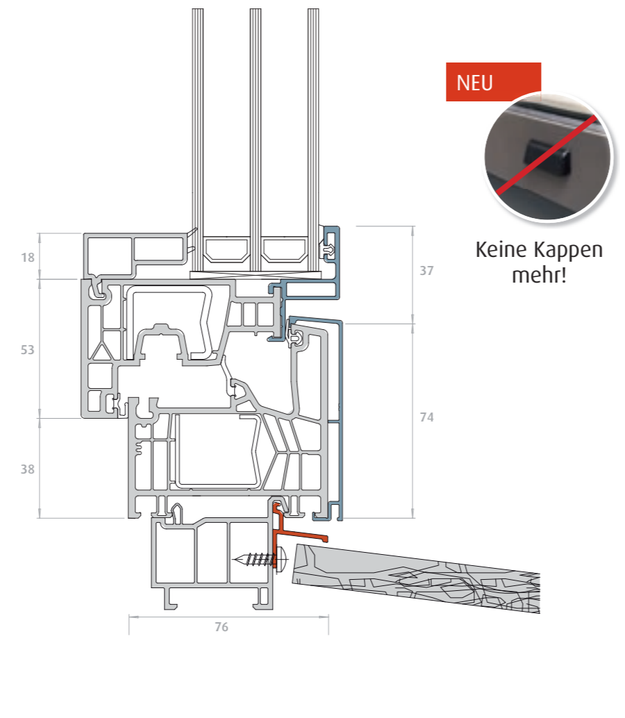
Steinbankanschluss
