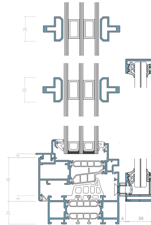
Glasabsturzicherung Typ2 und breiter Rahmen
