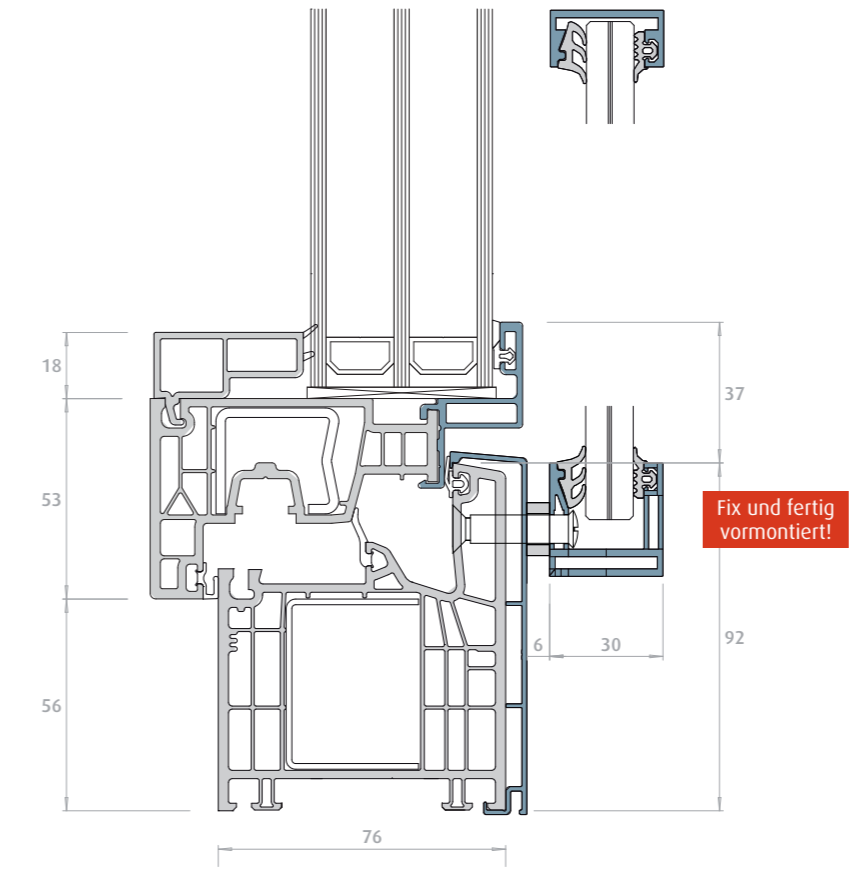
Glasabsturzicherung Typ2 und breiter Rahmen
